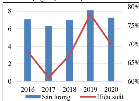
Sản lượng điện và hiệu suất của HND
